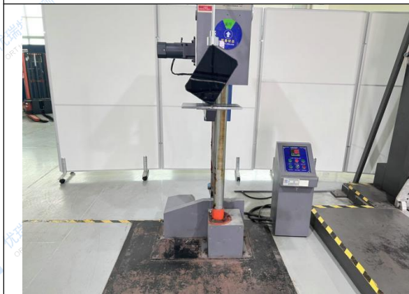
Fig.76 Test setup- Edge (9)
