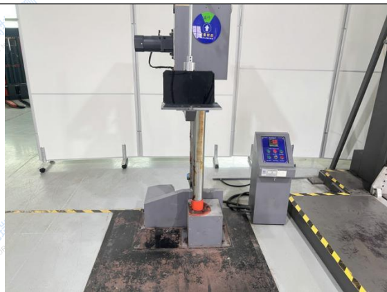
Fig.68 Test setup- Edge (1)
