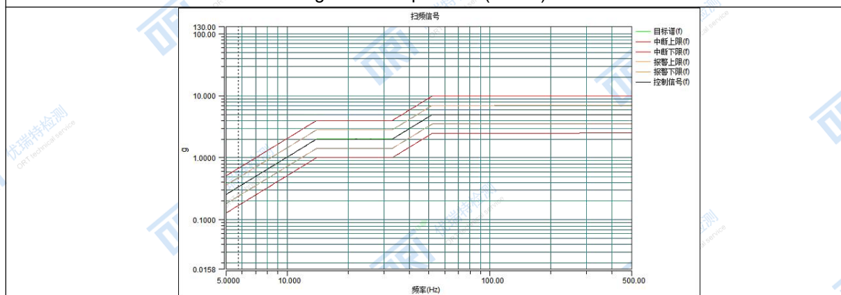
Fig.47 Test Spectrum (Z axis)
