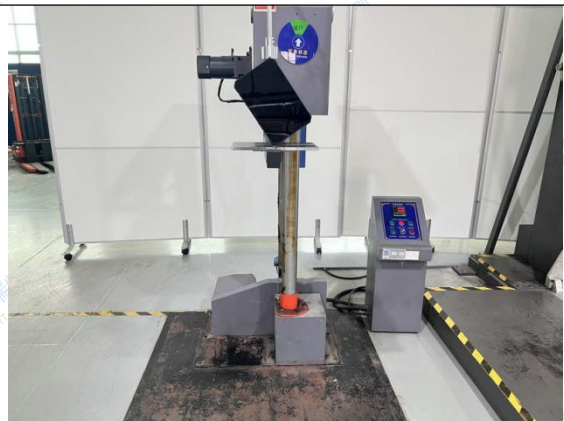
Fig.79 Test setup- Edge (12)
