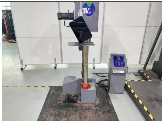
Fig.77 Test setup- Edge (10)
